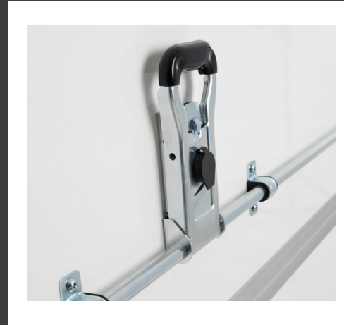
Verriegelung von außen mit Drehstangenverschluss
