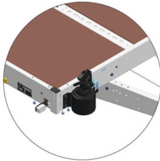
Position der Handpumpe bzw. Notpumpe bei Serienausstattung
