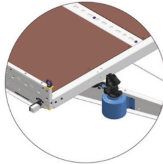
Position der Handpumpe bzw. Notpumpe optional
